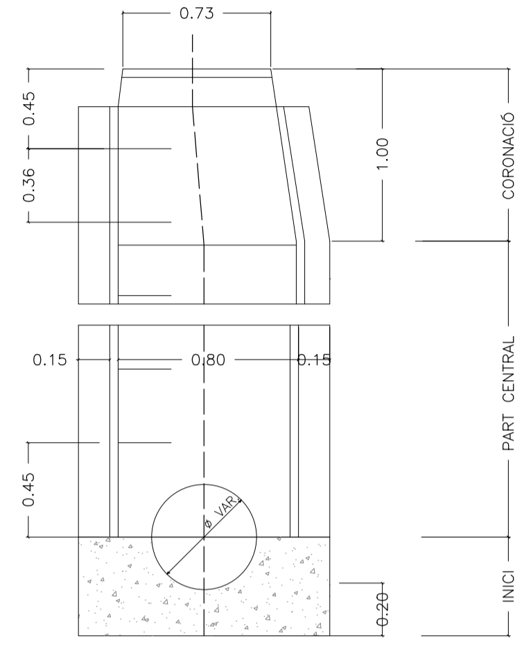
SECCIÓ C-C
