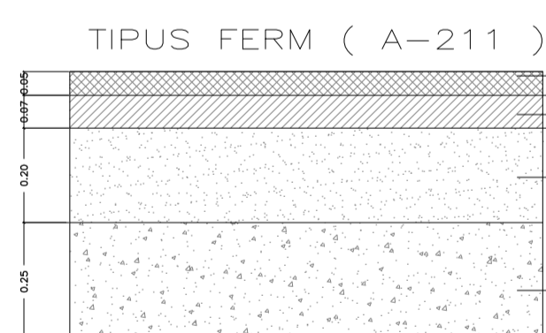
DETALL TIPUS DE FERM 1/20
