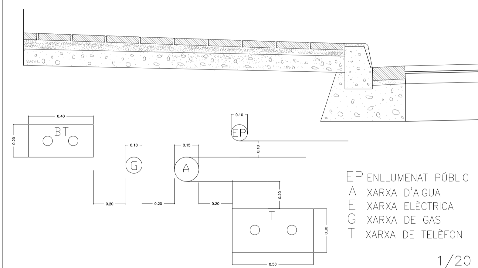
DETALL TIPUS DE FERM 1/20
