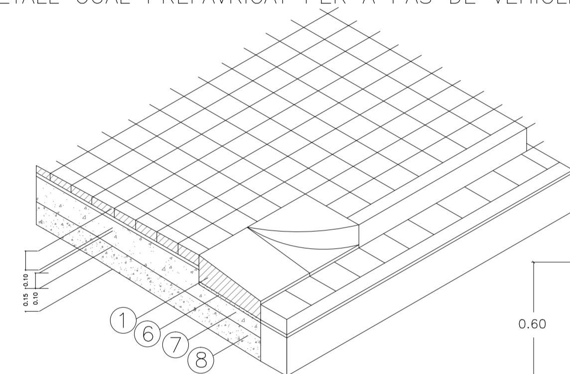
DETALL GUAL PREFABRICAT PER A PAS DE VEHICLES 1/25
