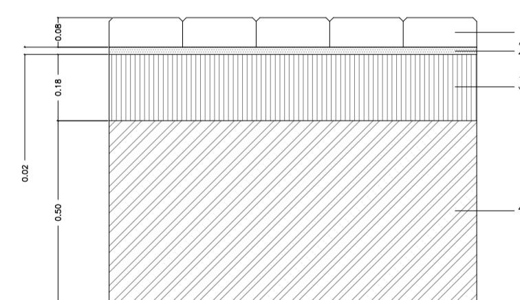
DETALL TIPUS DE FERM DE PECES DE FORMIGÓ DPF-1301 E 1/20
